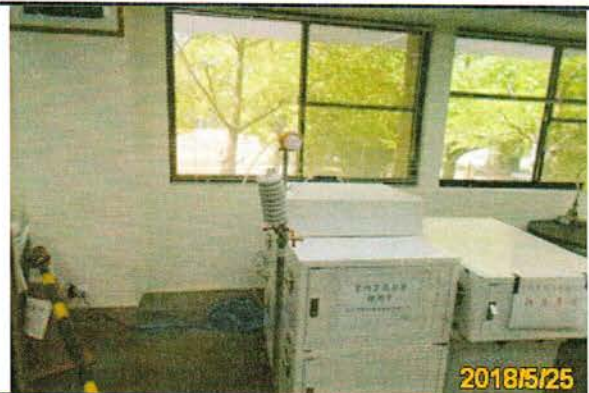
室內空氣品質~CO2、CO、溫度、濕度
